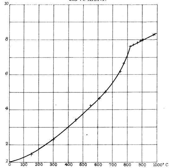
Pianoforte wire. Curve XXXVI.
